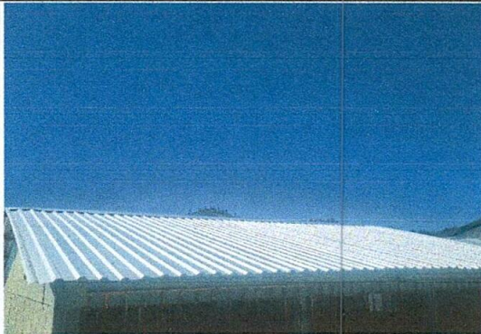
FOTO 3. SUSTITUCIÓN DE ESTRUCTURA DE SOPORTE DE MADERA
