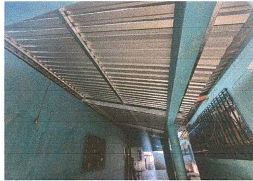
FOTO 2. SUSTITUCIÓN DE ESTRUCTURA DE SOPORTE DE MADERA
